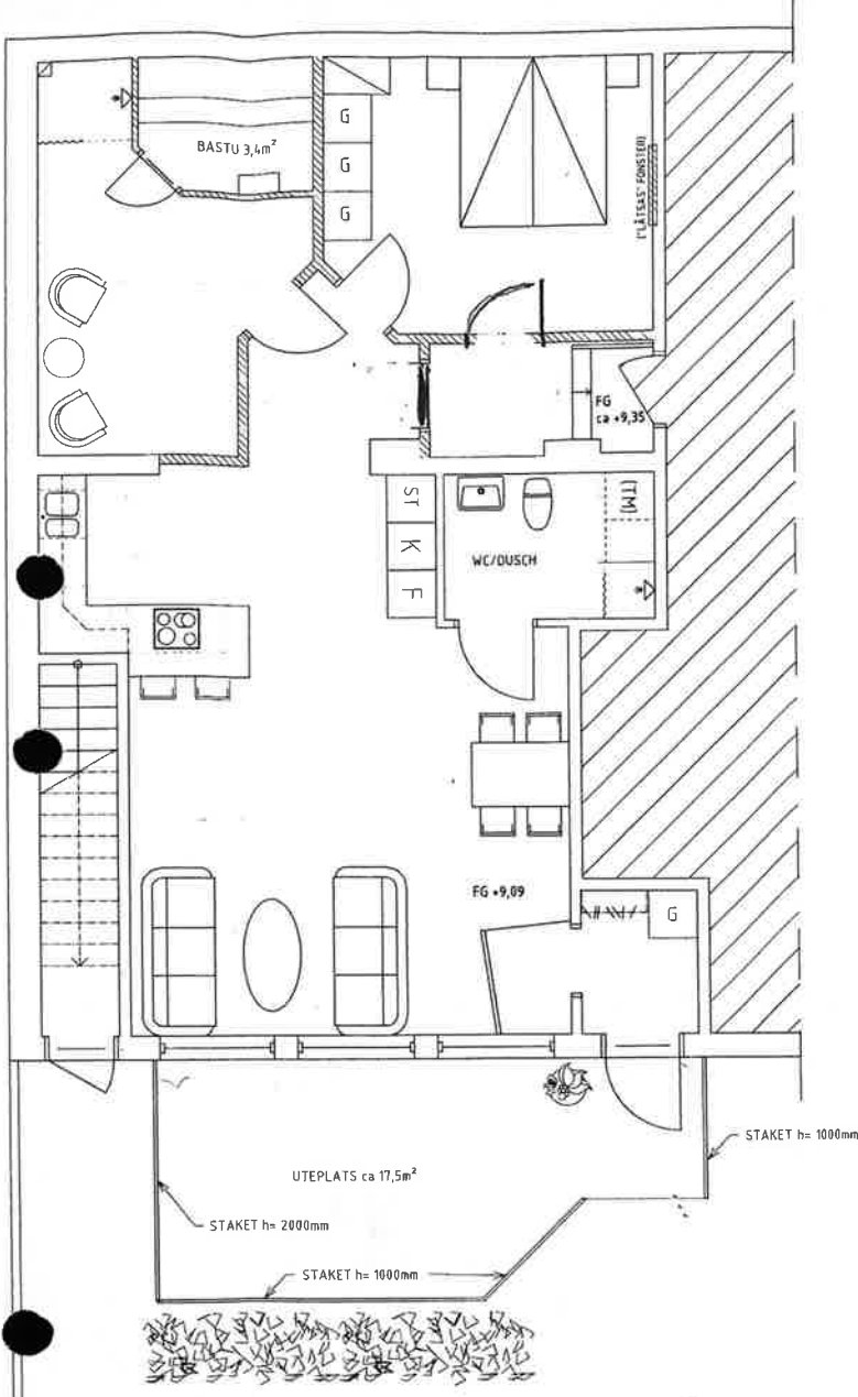
BLIV. PLAN 1:50
